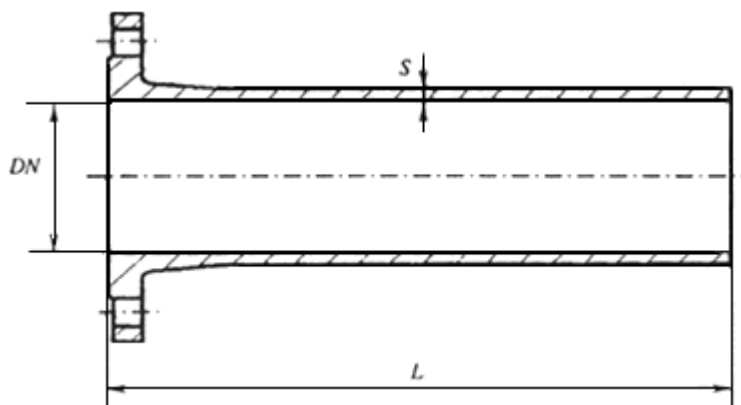
Патрубок компенсационный ПФРК 400 Б
