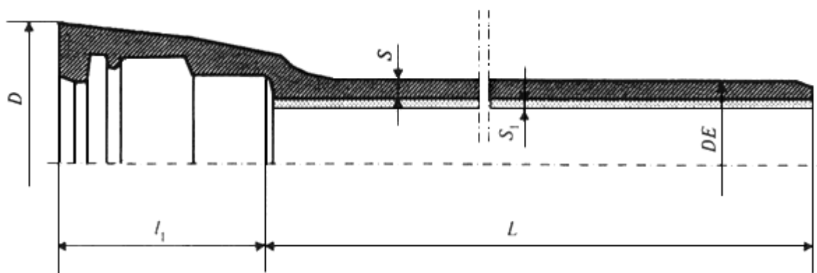
Рисунок А.1 - Труба раструбная под соединение "TYTON"
