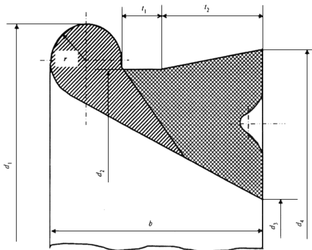
Рисунок А.8 - Уплотнительное резиновое кольцо под соединение "RJ"
