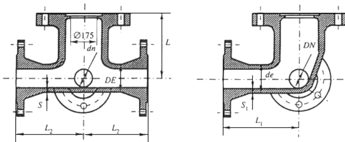
Рисунок Б.26 - Тройник фланцевый с пожарной подставкой
