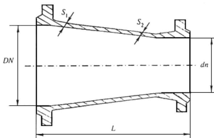
Переход ХРФ 200x100 (Т) Б
