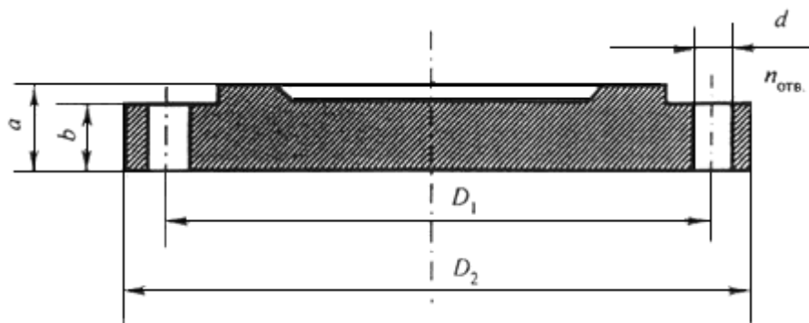
Рисунок Б.34 - Заглушка фланцевая
