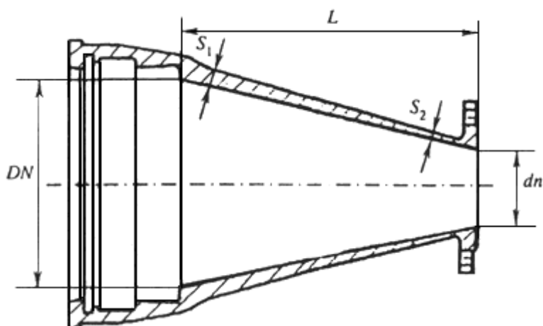
Переход ХРГ 200x100 (Т) Б
