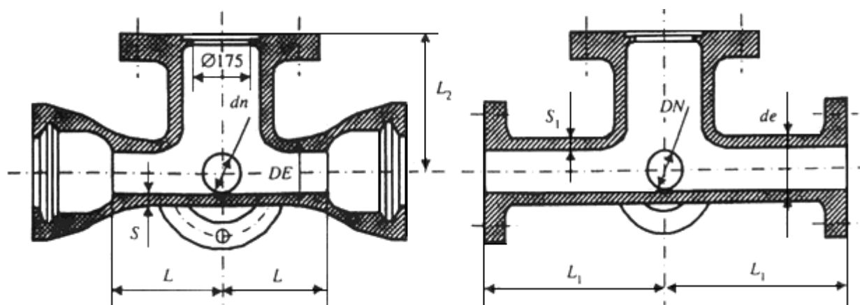
Крест КФ 600x400 Б
