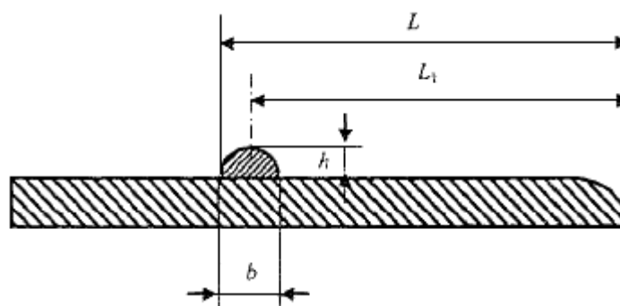
Рисунок 10.4 - Гладкий конец трубы с наплавленным валиком
