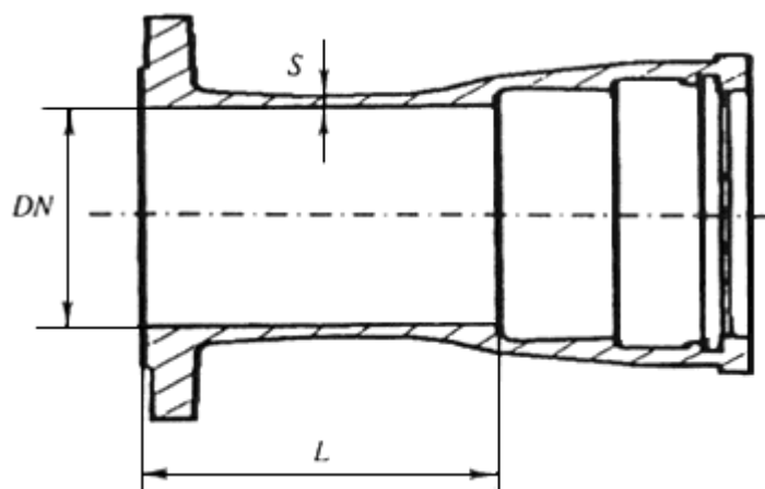
Переход ХР 200x100 (Т) А
