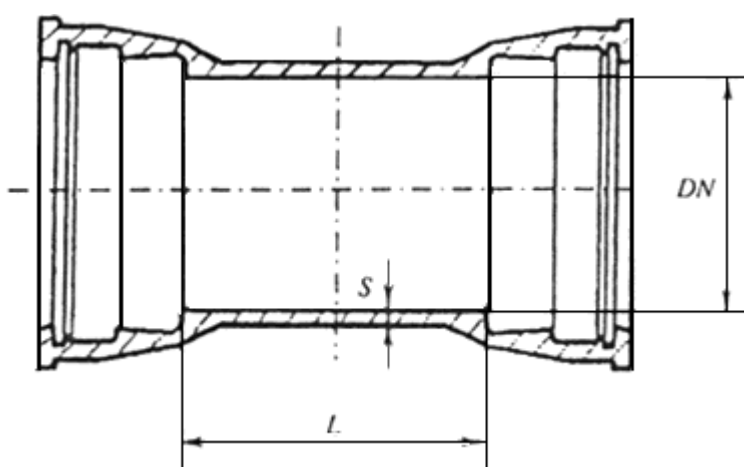
Патрубок ПФГ 200 Б
