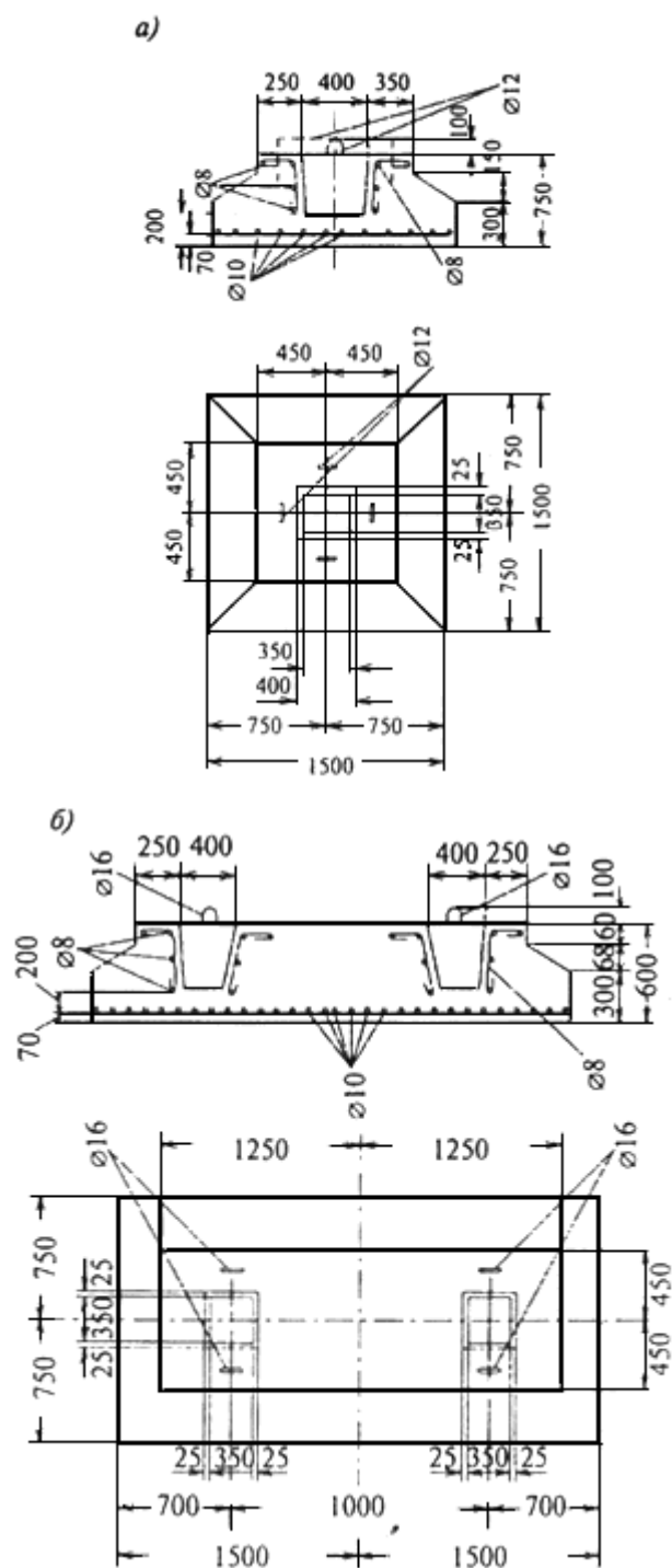
Рисунок 6.5 - Опорные железобетонные башмаки для труб диаметрами 400-500 мм под одну стойку (а), под две стойки (б)
