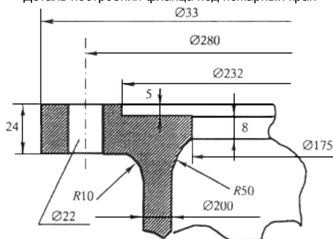
Деталь построения фланца под пожарный кран
