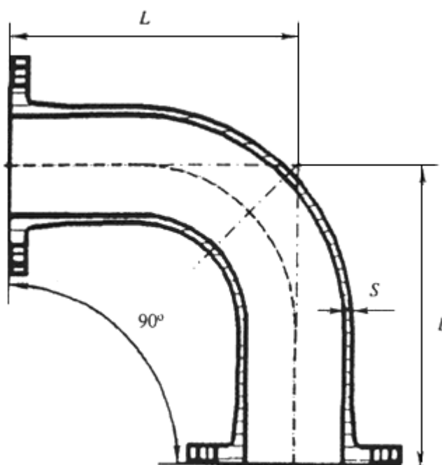
Рисунок Б.8 - Колено фланцевое
