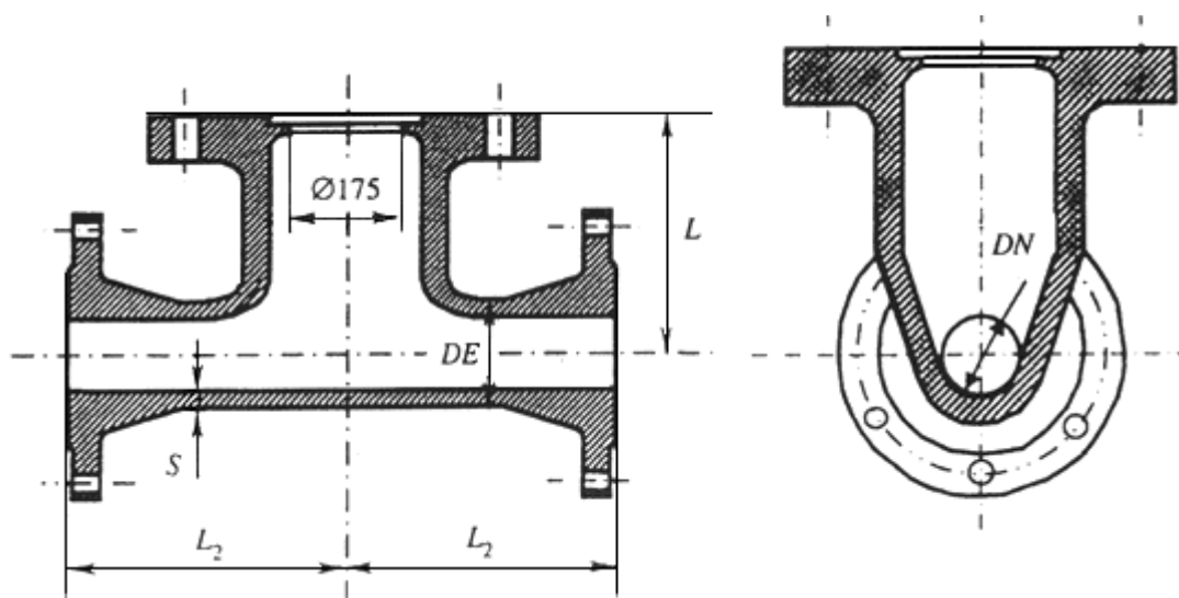
Рисунок Б.35 - Пожарная подставка фланцевая
