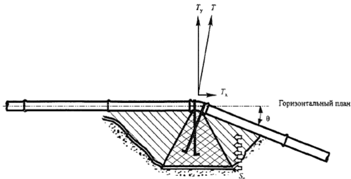
Рисунок 11.3 - Гравитационный блок для вертикальных изгибов
