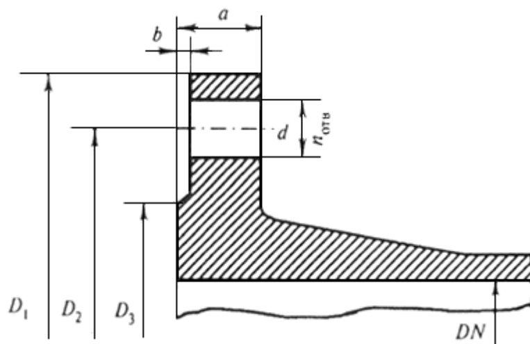
Рисунок Б.3 - Фланец
