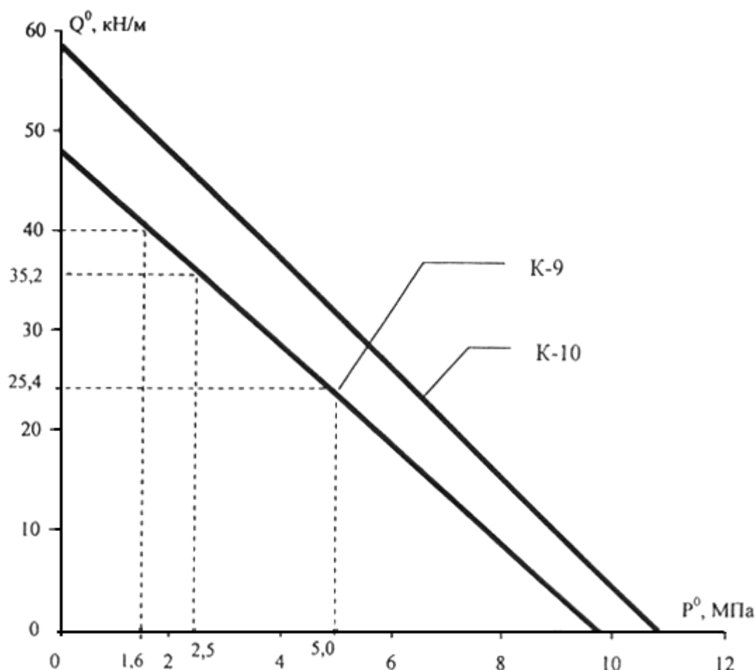
Рисунок 5.6 - Графики прочности труб диаметром 600 мм классов К-9 и К-10
