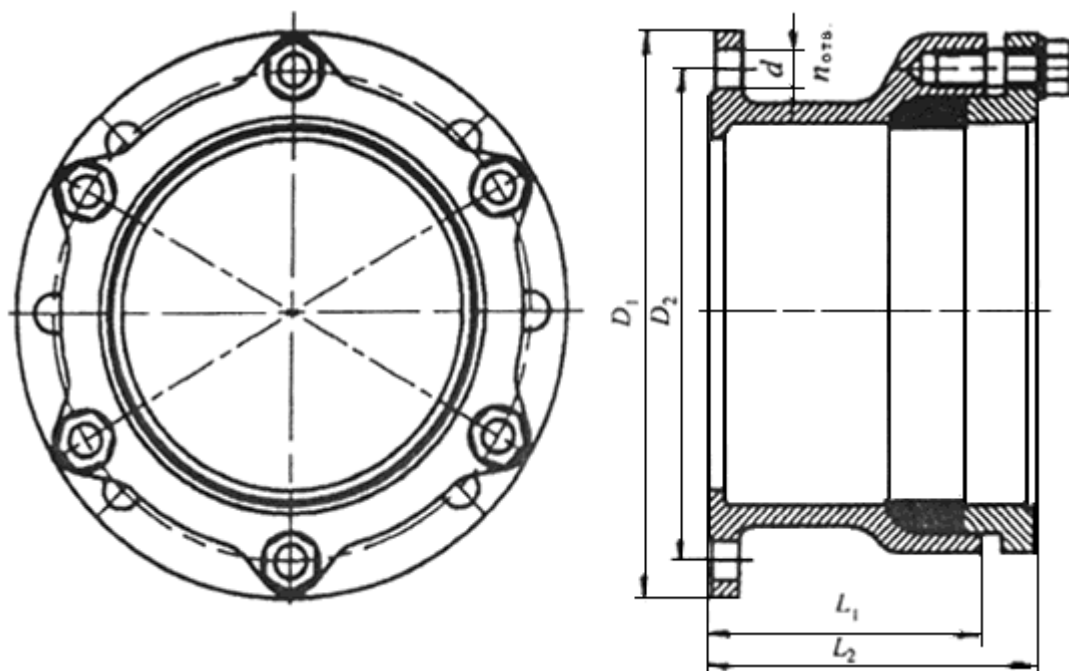
Рисунок Б.18 - Патрубок фланец-раструб компенсационный
