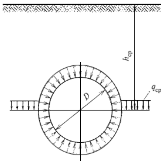
Рисунок 7.1 - Среднее давление грунта на подземный трубопровод
