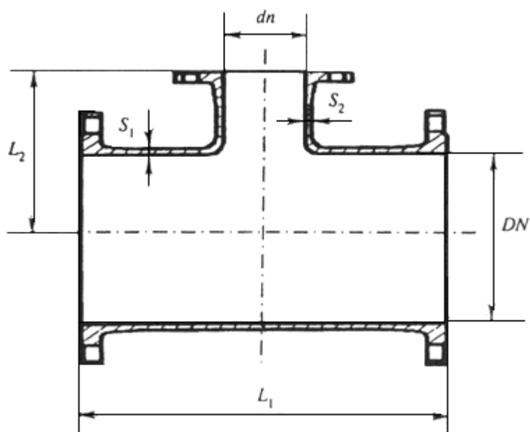
Тройник TP 400x150 (Т) А
