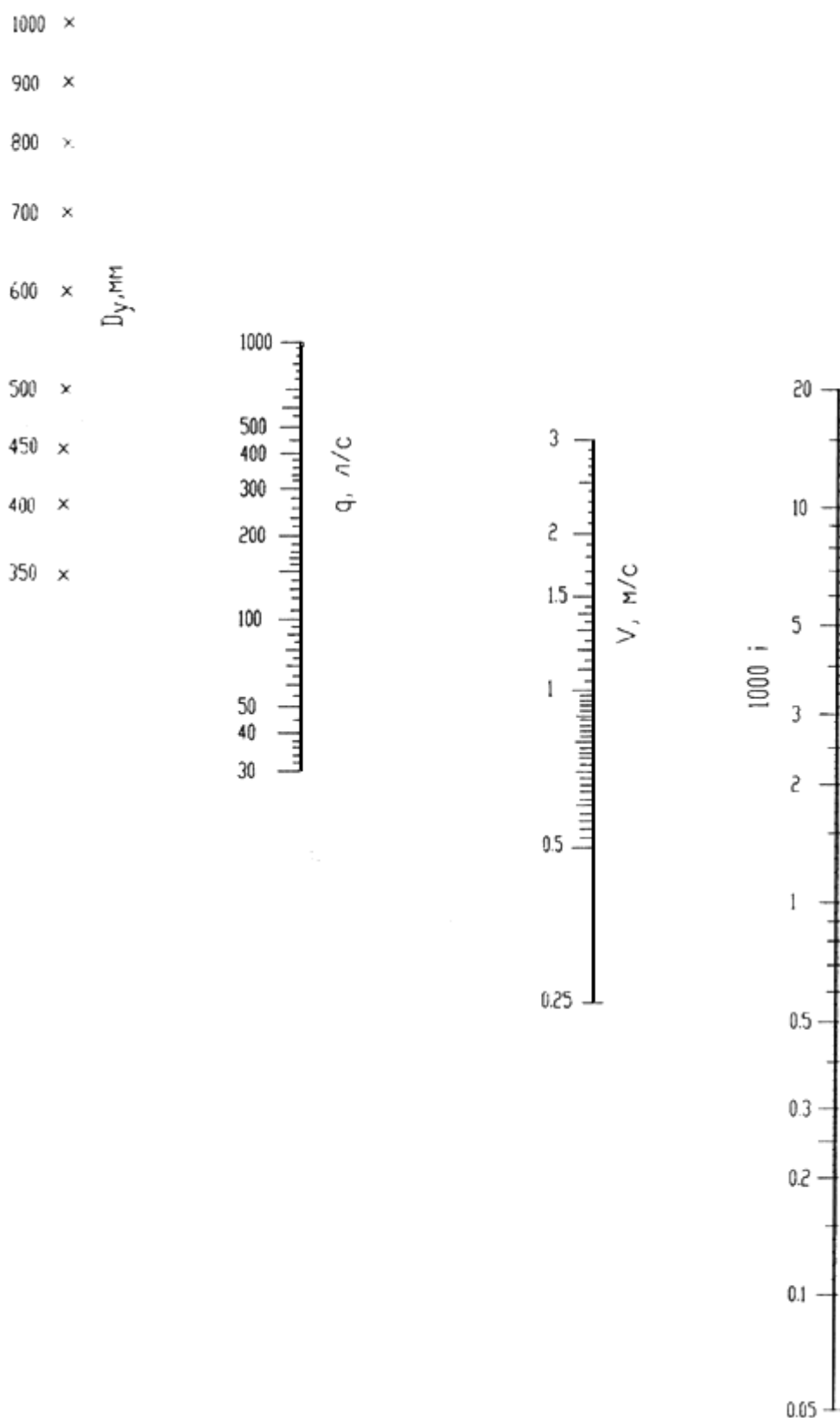
Рисунок 5.1 - Номограмма для приближенных гидравлических расчетов напорных трубопроводов диаметрами 100-300 мм из высокопрочных труб из чугуна с шаровидным графитом класса К-9 с внутренним цементно-песчаным покрытием
