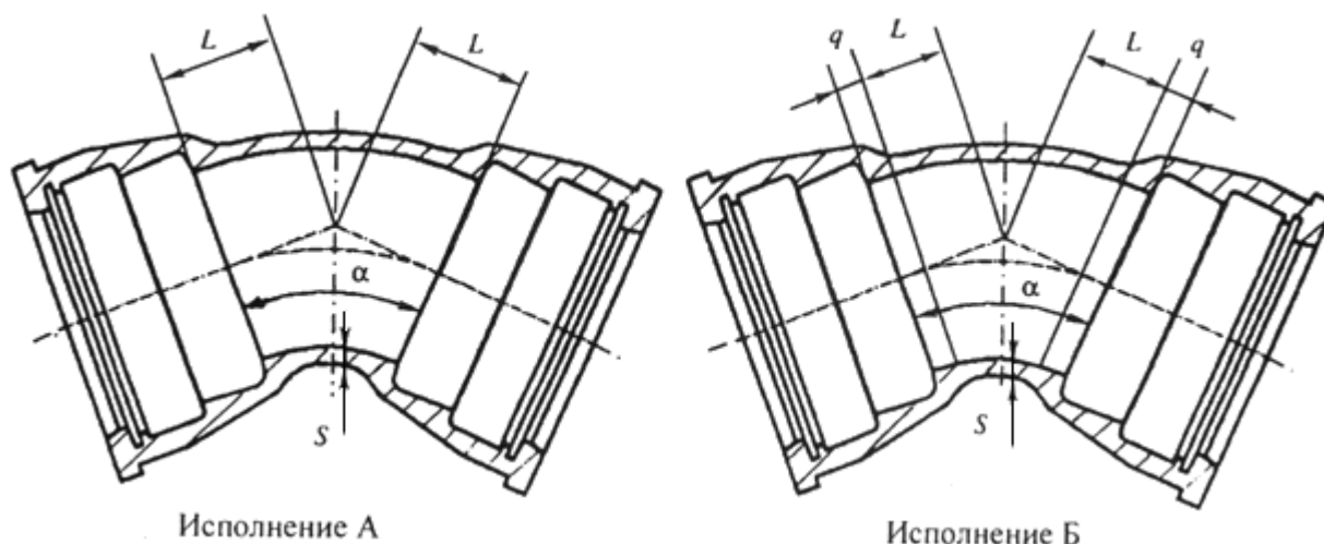
Рисунок Б.11 - Отвод раструбный
