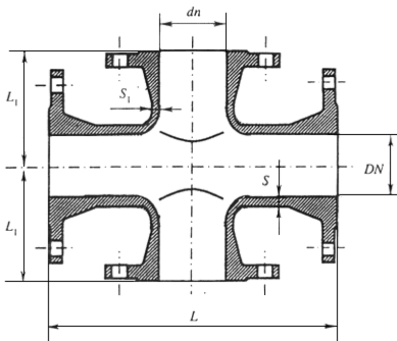
Крест КР 600x400 (Т) Б
