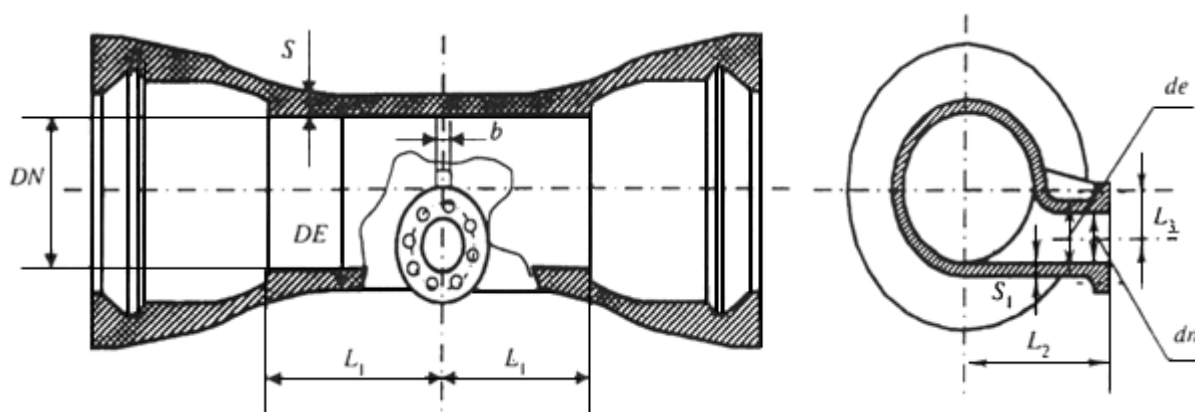
Рисунок Б.22 - Выпуск раструбный
