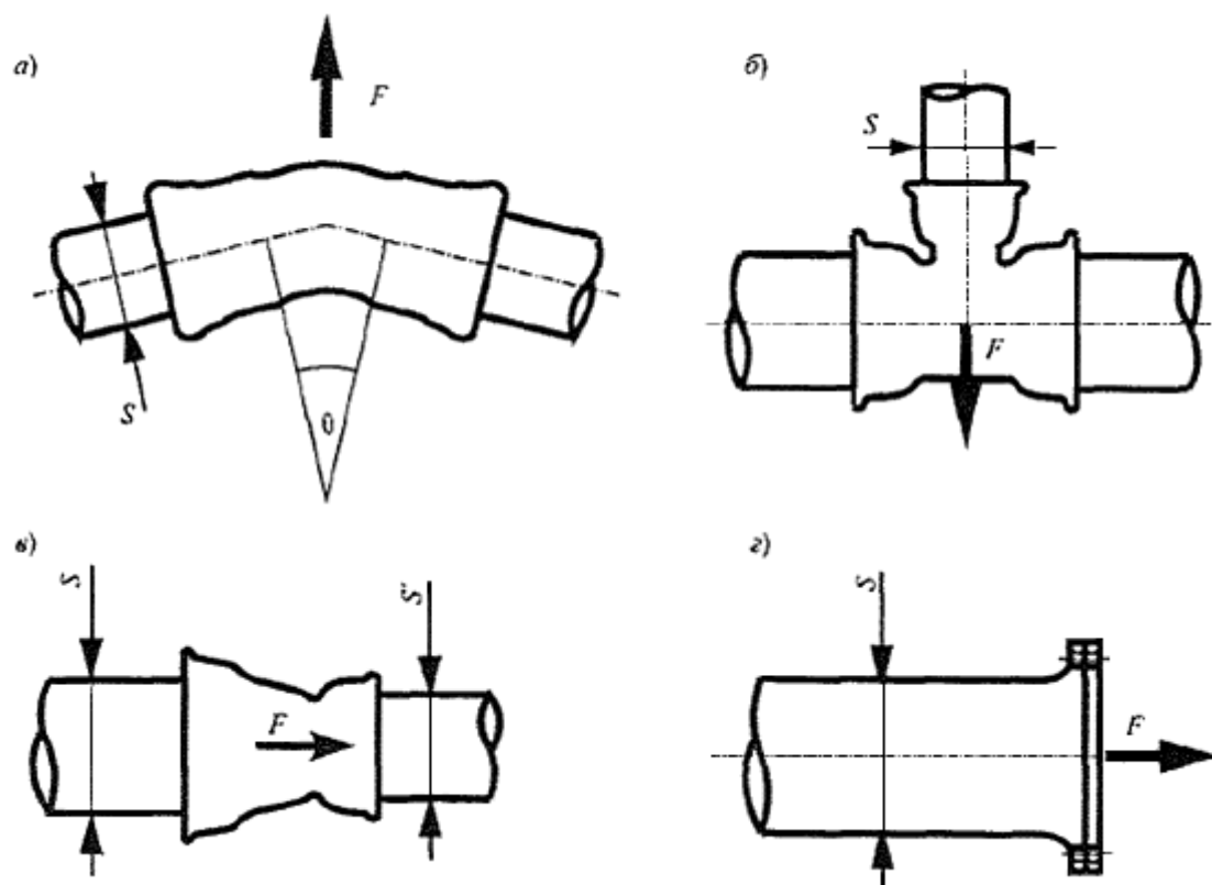
Рисунок 11.2 - Примеры схем конструкций соединений труб
