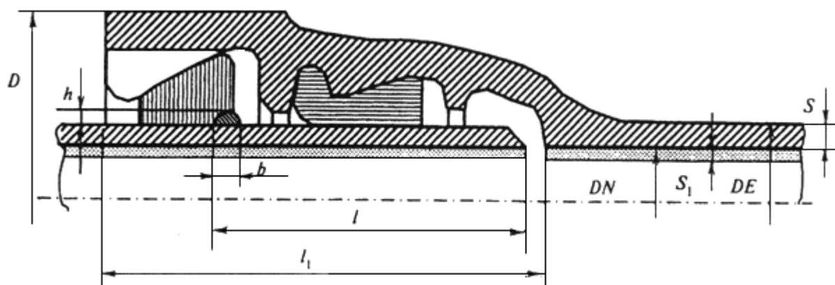
Рисунок Б.1 - Раструбное соединение типа "RJ"
