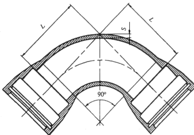
Рисунок Б.9 - Колено раструбное
