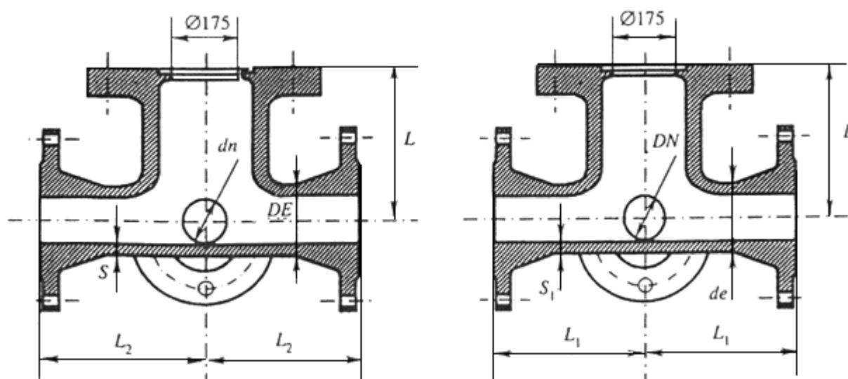
Крест ППКРФ 200x150 (Т) Б
