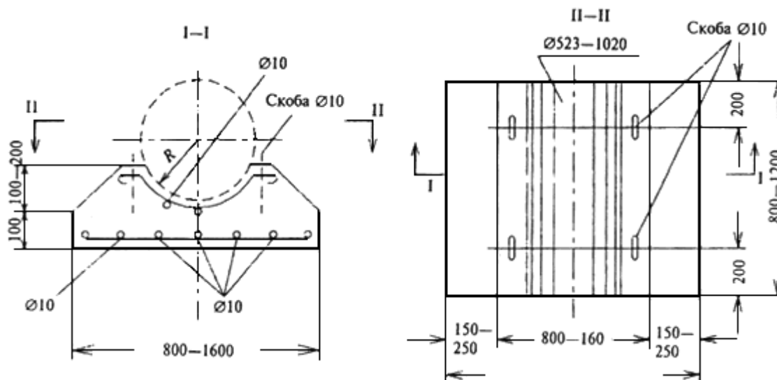
Рисунок 6.4 - Плитная опора с ложем для укладки трубопровода
