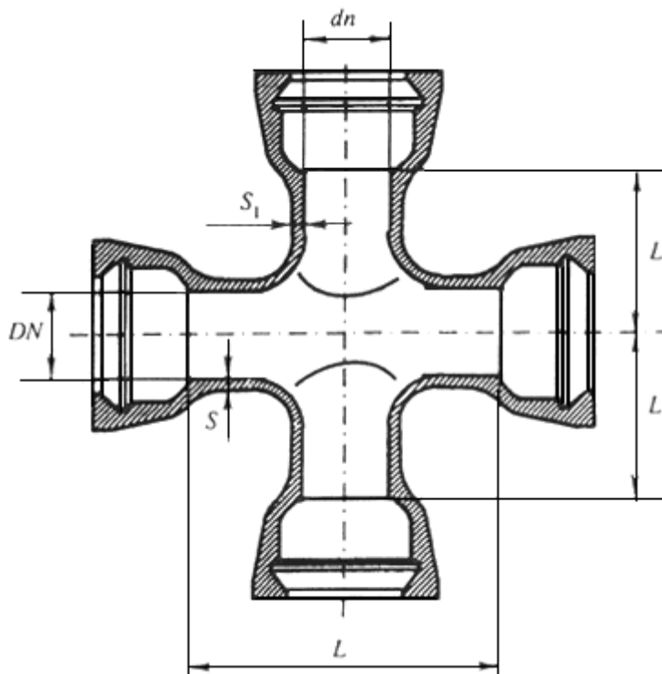
Крест КРФ 400x200 (Т) Б
