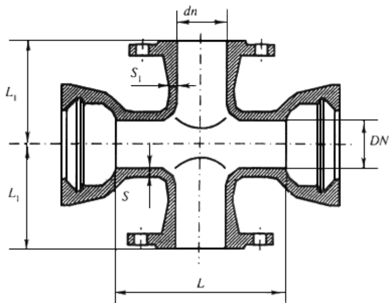
Рисунок Б.27 - Крест раструб-фланец
