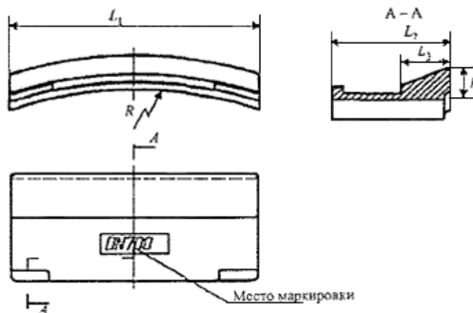
Рисунок 10.3 - Стопорные элементы под соединение типа "RJS"
