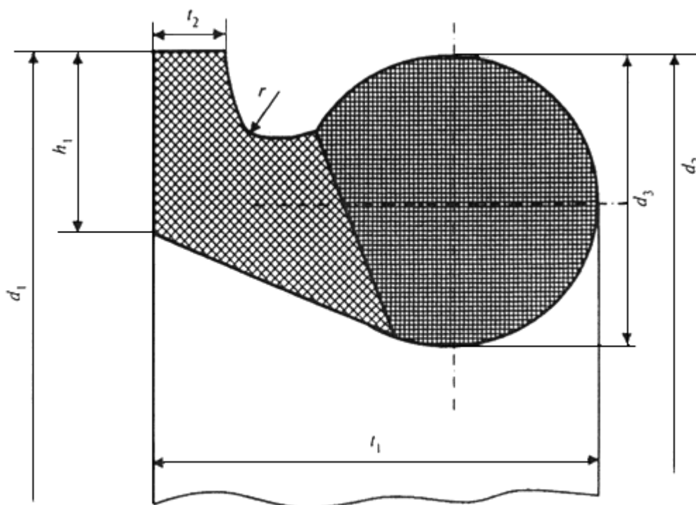
Рисунок А.7 - Уплотнительное резиновое кольцо под соединение "TYTON"
