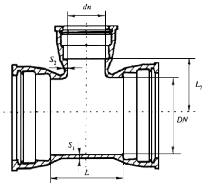
Рисунок Б.5 - Тройник раструбный
