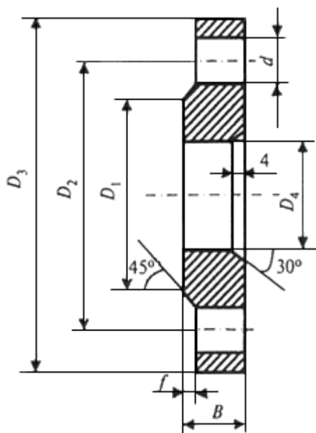
Рисунок А.4 - Фланец из высокопрочного чугуна
