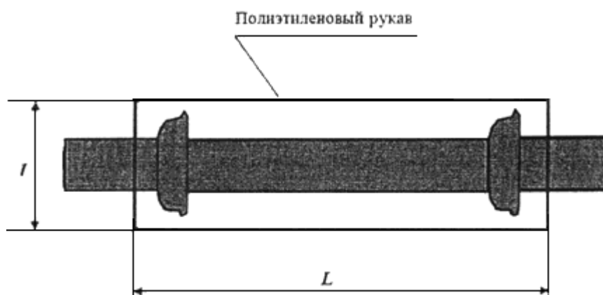
Рисунок 5.7 - Полиэтиленовый рукав для труб
