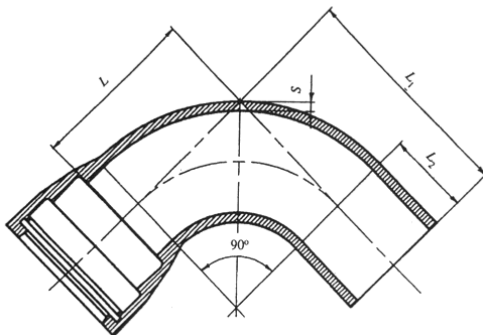
Рисунок Б.7 - Колено раструб-гладкий конец
