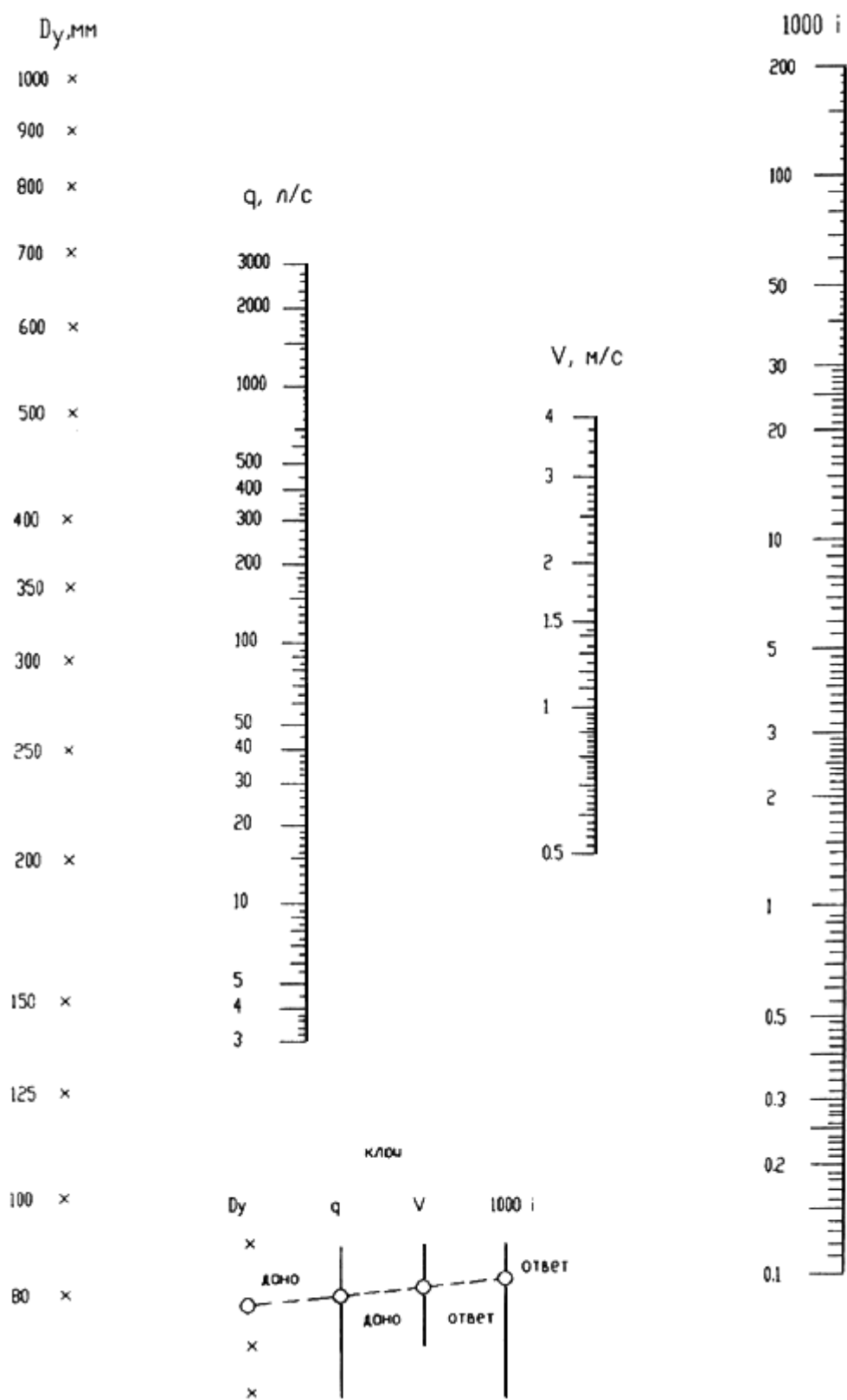
Рисунок 5.3 - Номограмма для приближенных гидравлических расчетов напорных трубопроводов из высокопрочных труб из чугуна с шаровидным графитом класса К-9 без покрытия
