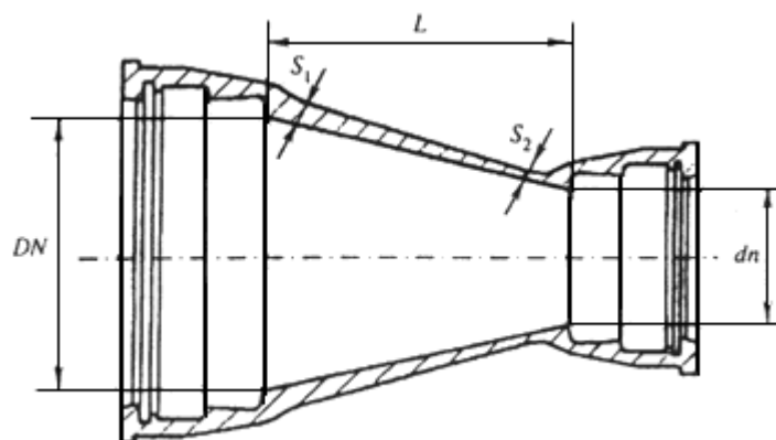
Рисунок Б.16 - Переход раструбный
