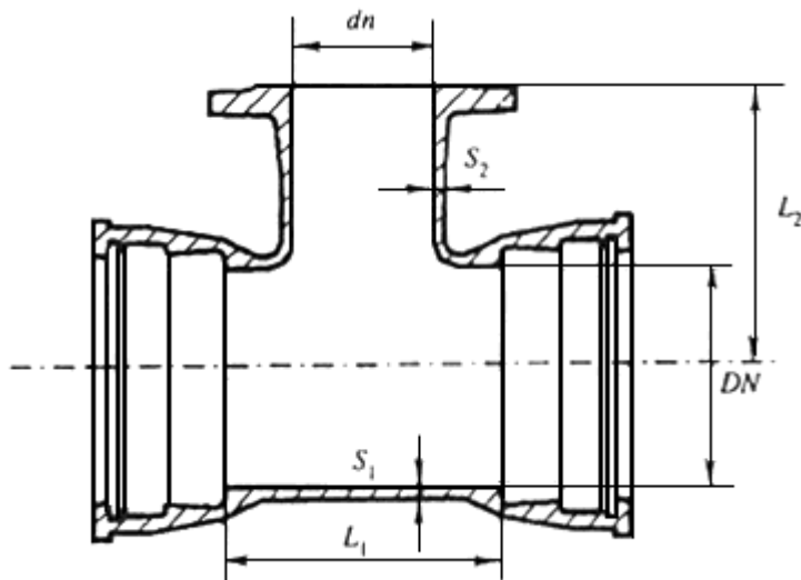
Рисунок Б.4 - Тройник раструб-фланец
