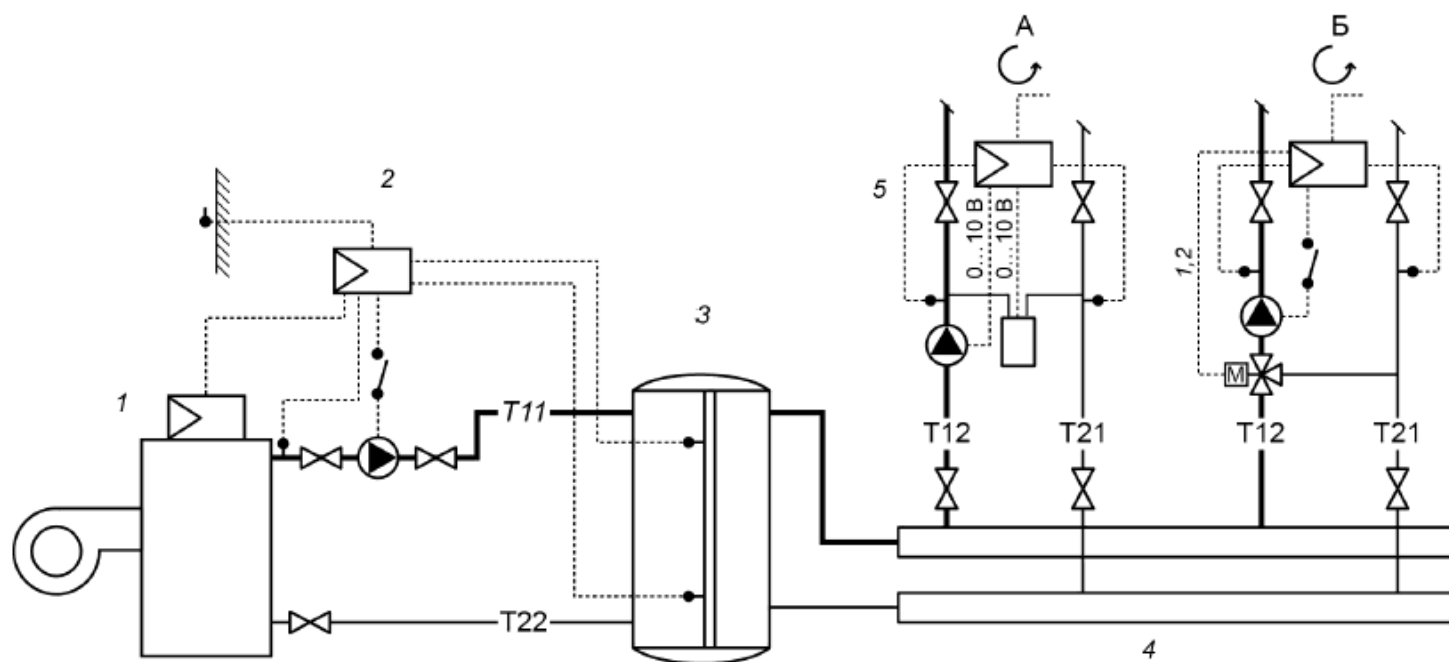
1 - котельная установка; 2 - контроллер управления источника 1; 3 - буферная емкость теплоносителя; 4 - распределительный коллектор; 5 - контур теплоснабжения: А - жилых помещений, Б - мест общего пользования
