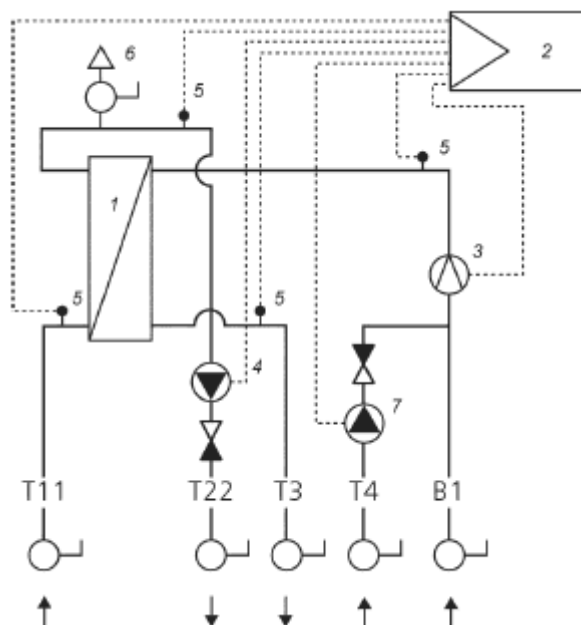
Рисунок 7.13 - Гидравлическая схема КТП для обеспечения локального ГВС
