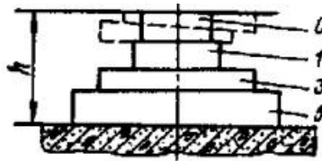
Рис. 6. Пирамидальный пакет подкладок:
