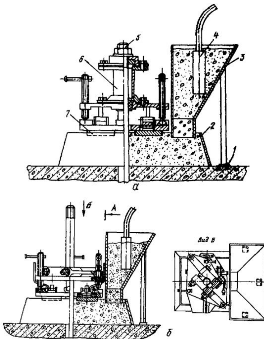
Устройство для установки опорных элементов на фундаменте:
