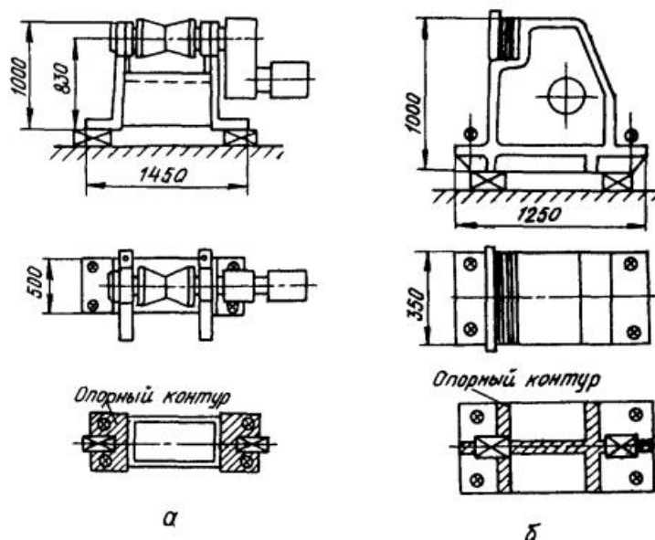
Расположение опорных элементов при выверке:
