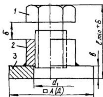
Рис. 2. Винтовая подкладка:
