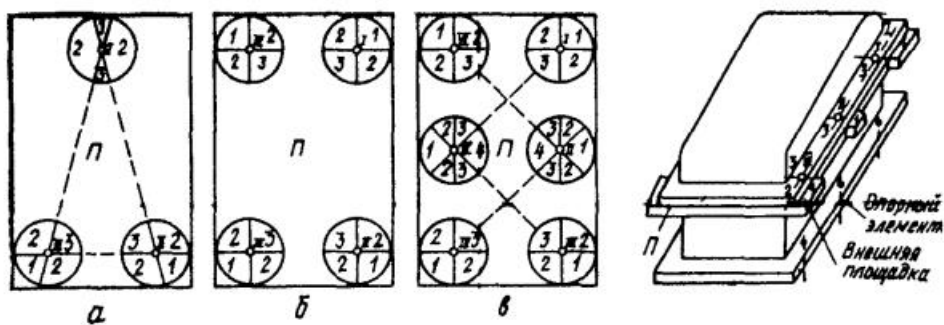
Рис. 1. Схема рационального расположения площадок установки измерительных средств:
