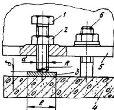
Рис. 2. Выверка оборудования с помощью регулировочных винтов:
