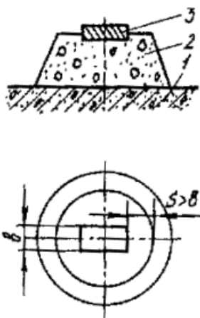
Рис. 8. Бетонная опора с металлической пластиной:
