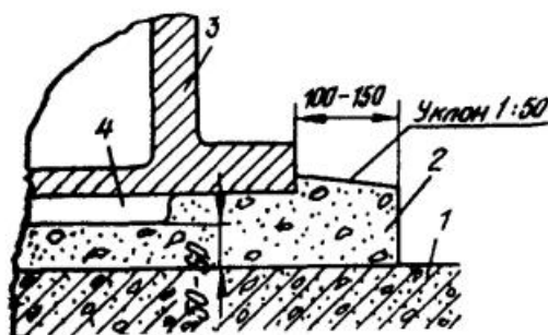
Рис. 9. Схема подливки оборудования:
