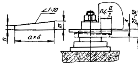
Рис. 7. Клиновые подкладки
