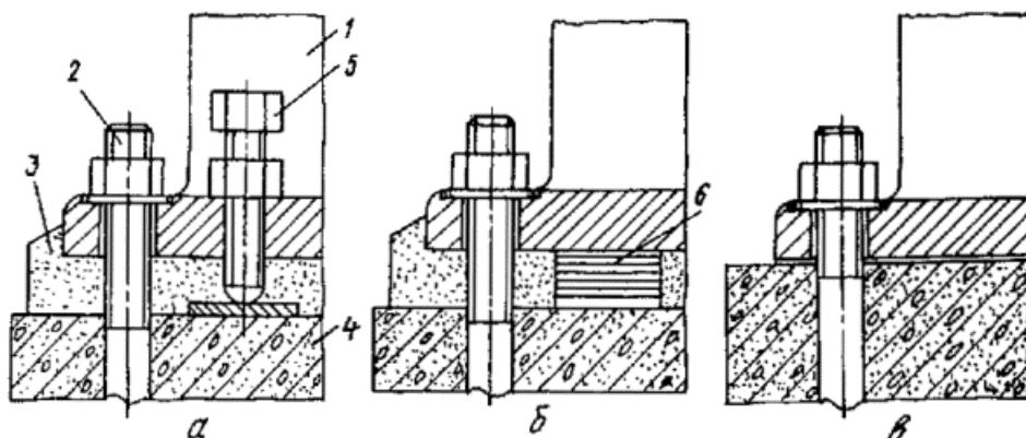
Рис. 1. Типы соединений "оборудование-фундамент":
