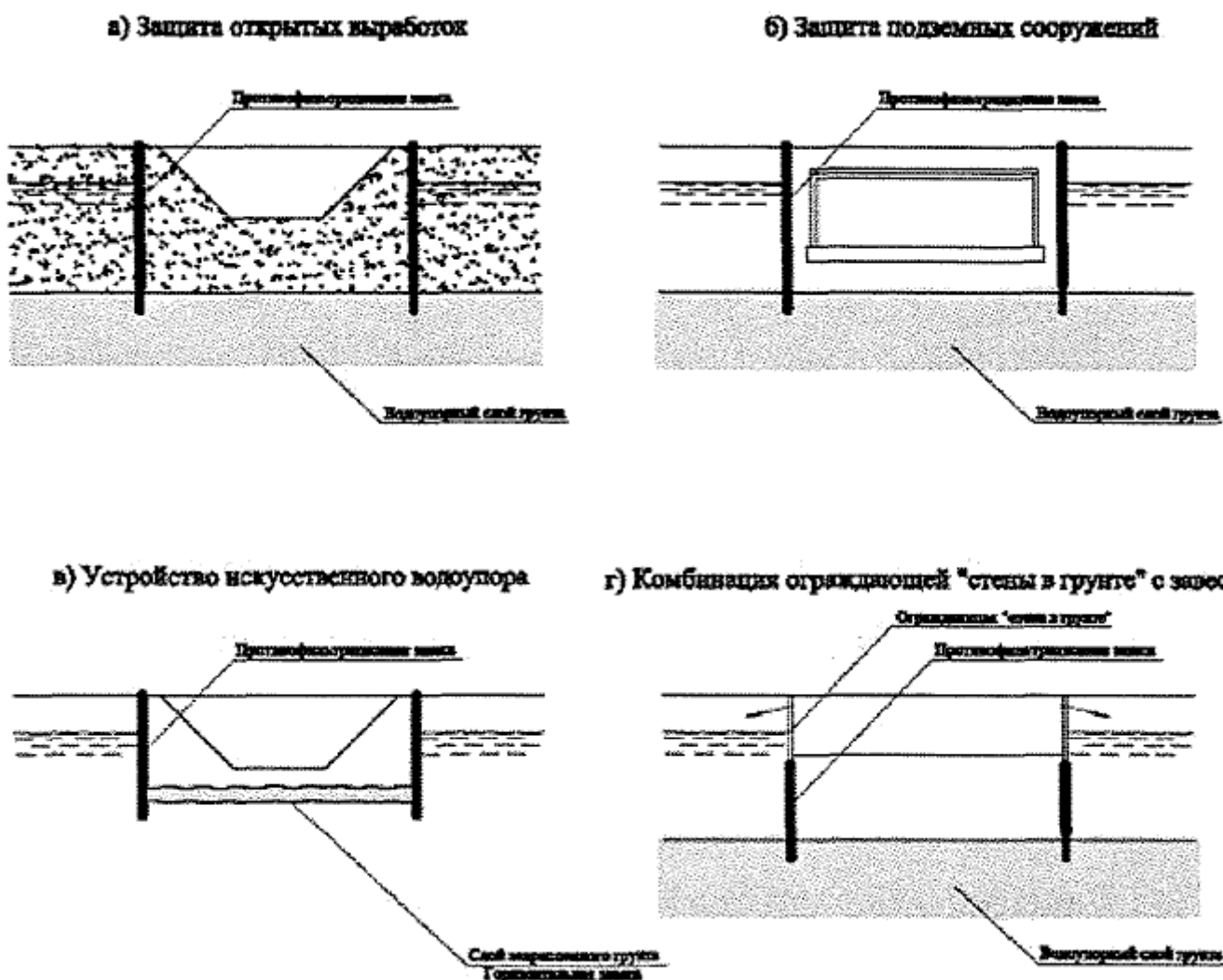
а) - защита открытых выработок; б) - защита подземных сооружений; в) - устройство искусственного водоупора; г) - комбинация ограждающей "стены в грунте" с завесой
