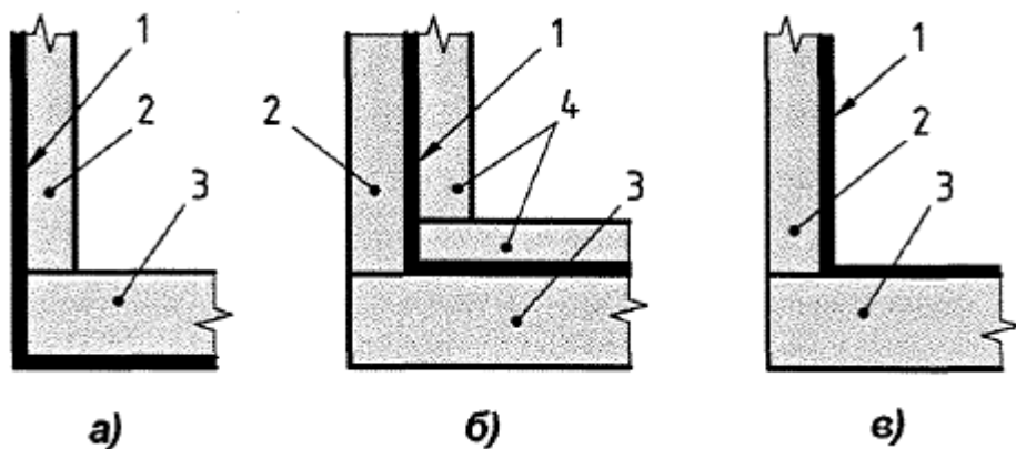
а) наружная гидроизоляция; б) гидроизоляция сэндвичного типа; в) внутренняя гидроизоляция 1 - гидроизоляционный материал; 2 - наружная стена сооружения; 3 - фундаментная плита; 4 - прижимные конструкции
