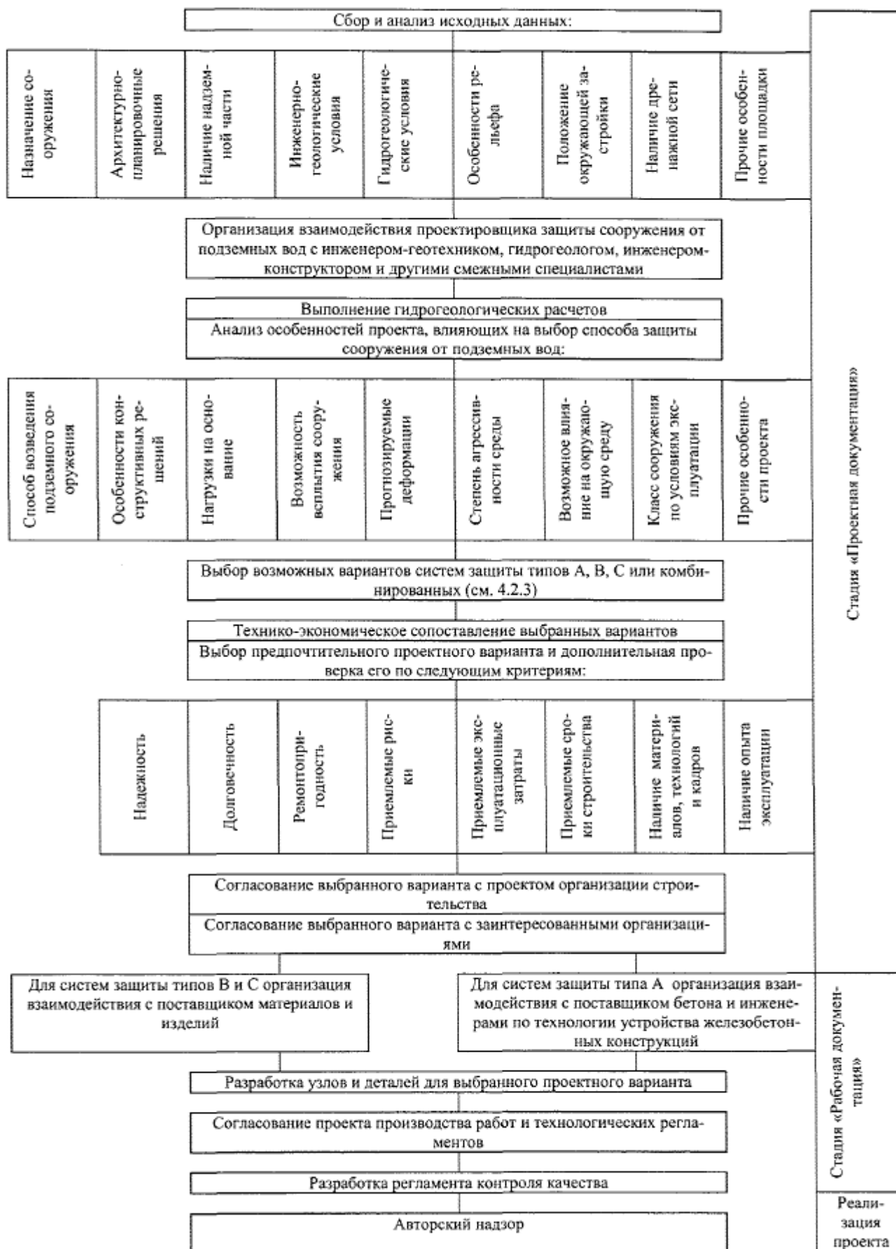
Рисунок 5.1 - Схема последовательности этапов проектирования защиты сооружения от подземных вод
