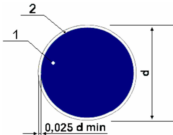
d - диаметр круга; 1 - основная поверхность; 2 - кант Рисунок 3 - Основа цветографического изображения и соотношение размеров предписывающих знаков безопасности
