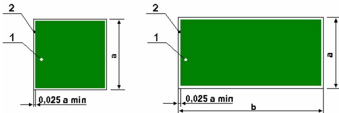
a, b - стороны квадрата и прямоугольника ( 2a = b ); 1 - основная поверхность; 2 - кант Рисунок 5 - Основа цветографического изображения и соотношение размеров эвакуационных знаков безопасности и знаков безопасности медицинского и санитарного назначения
