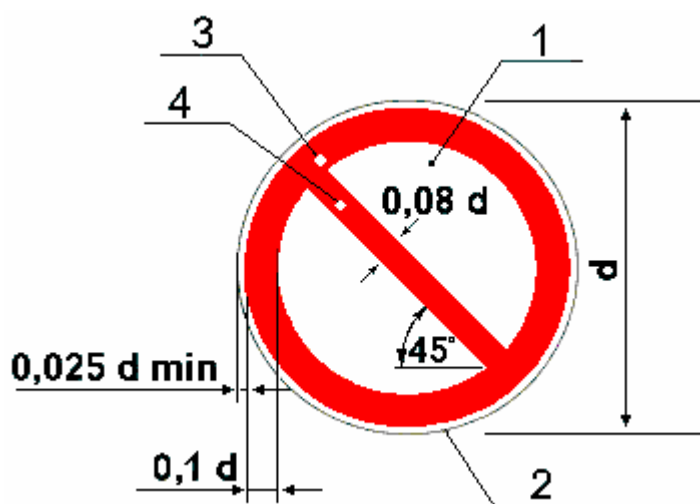
d - диаметр круга; 1 - основная поверхность; 2 - кант; 3 - кайма; 4 - поперечная полоса Рисунок 1 - Основа цветографического изображения и соотношение размеров запрещающих знаков безопасности
