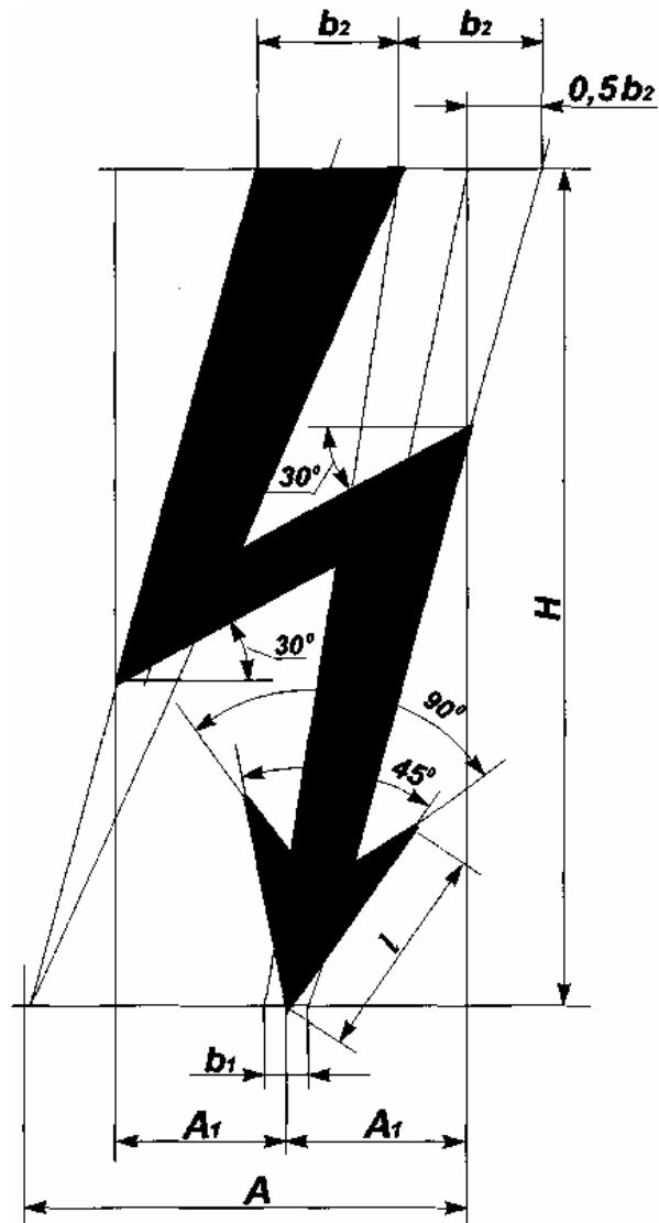
Рисунок Л.1 — Графический символ электрического напряжения
