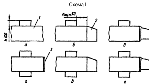
Схемы образования узлов ответвлений прямоугольного сечения
