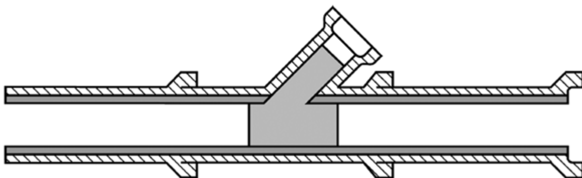
Этап 3. Сдвиг пакера, извлечение оборудования
