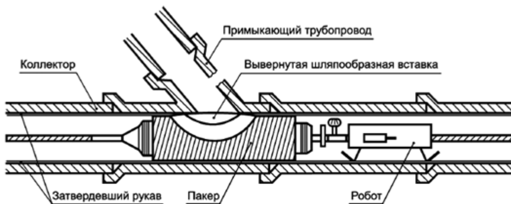
Этап 1. Positionирование пакера со шляпообразной вставкой
