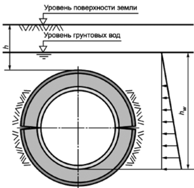
Рисунок 3* - Система "старая труба-грунт". Класс состояния 2
