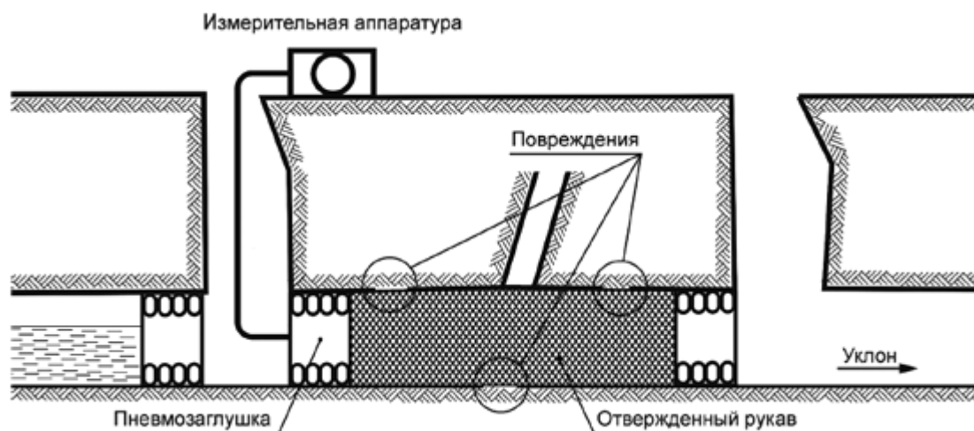
Рисунок 15* - Монтаж гибких полимерных рукавов, отверждаемых УФ-излучением.
