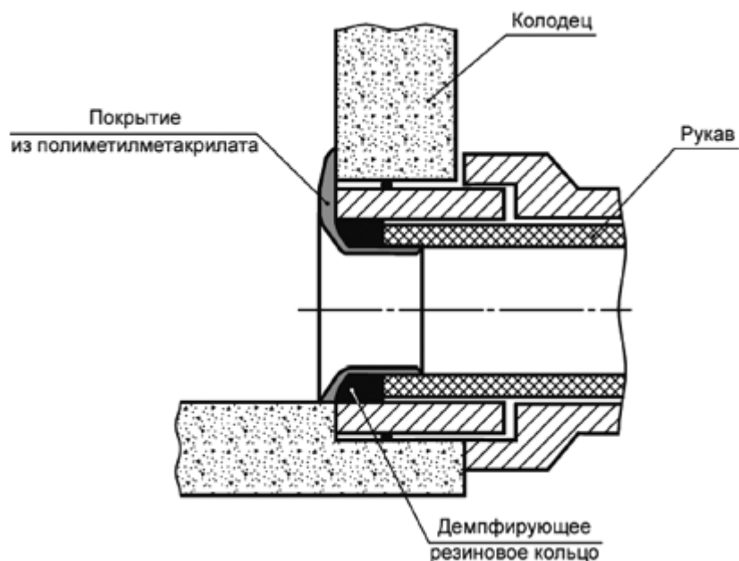
Рисунок 22* - Устройство примыкания с применением манжет на основе полиметилметакрилата
