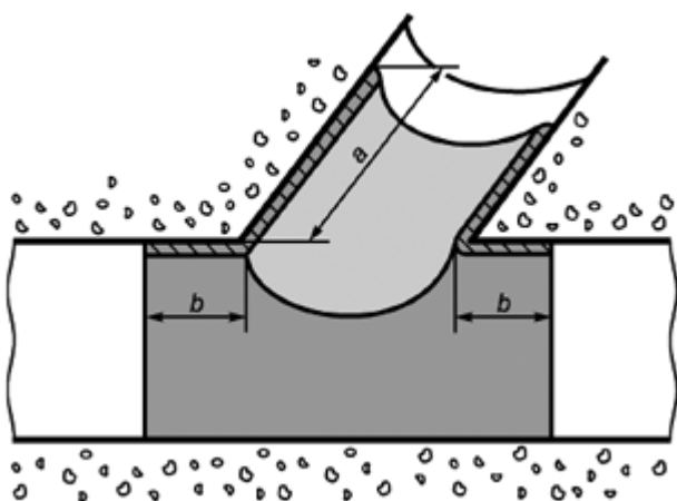
Рисунок 20* - Т-образная манжета
