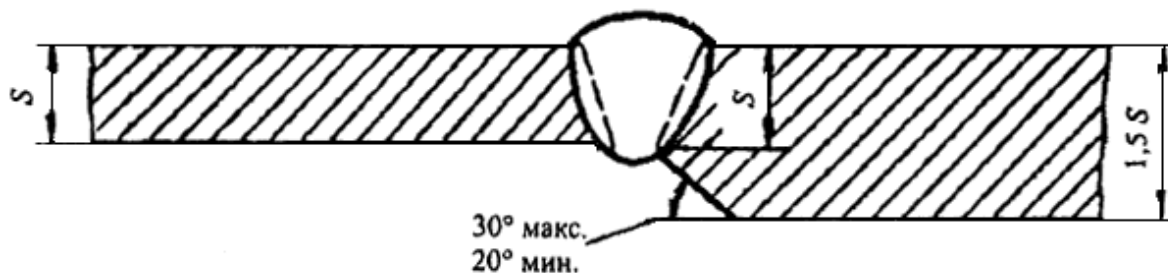
Рисунок 1 - Конструктивные размеры разделки кромок и сварных швов разнотолщинных труб (до 1,5 толщины стенки)
