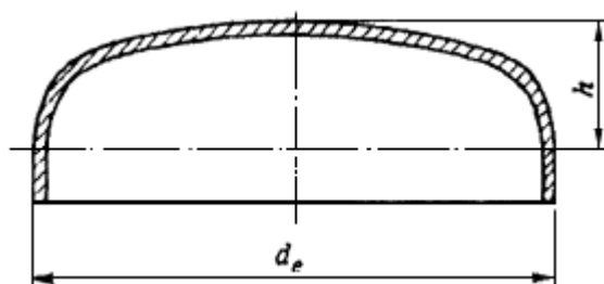
Рисунок А.3 - Заглушка эллиптическая
