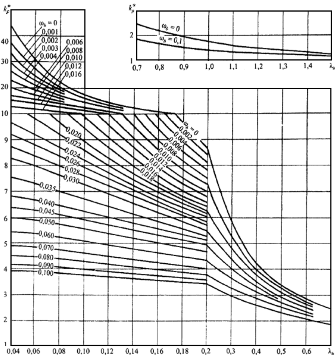
Рисунок 1 - График для определения значений коэффициента k_p^*
