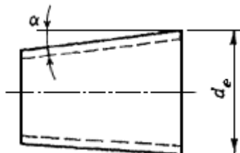
Рисунок А.2 - Концентрический переход
