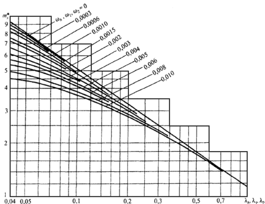
Рисунок 2 - График для определения значений коэффициента m_s^*
