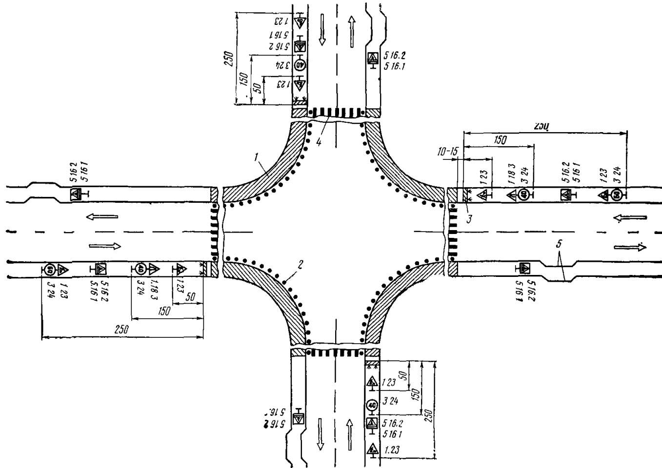
Рис. 3.14. Организация движения и ограждение мест дорожных работ, выполняемых на обочинах пересечения в одном уровне: 1 — зона работ; 2 — направляющие конусы; 3 — ограждающие барьеры; 4 — существующие пешеходные переходы, закрываемые на период дорожных работ; 5 — автобусные остановки, перенесенные из зоны дорожных работ
