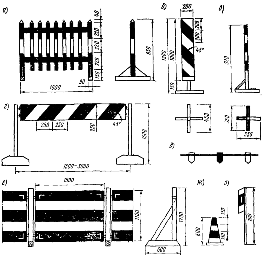
Рис. 4.2. Ограждения и направляющие устройства:
