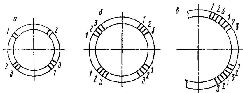
Рис.3. Схема вырезки образцов для механических испытаний а - трубы диаметром до 400 мм включительно; б - трубы диаметром от 100 мм до 1000 мм; в - трубы диаметром 1000 мм и более; 1 - образец для испытания на растяжение (ГОСТ 6996-66, тип XII или XIII); 2 - образец на изгиб корнем шва наружу
